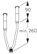
SG 6658 V-Hanger
